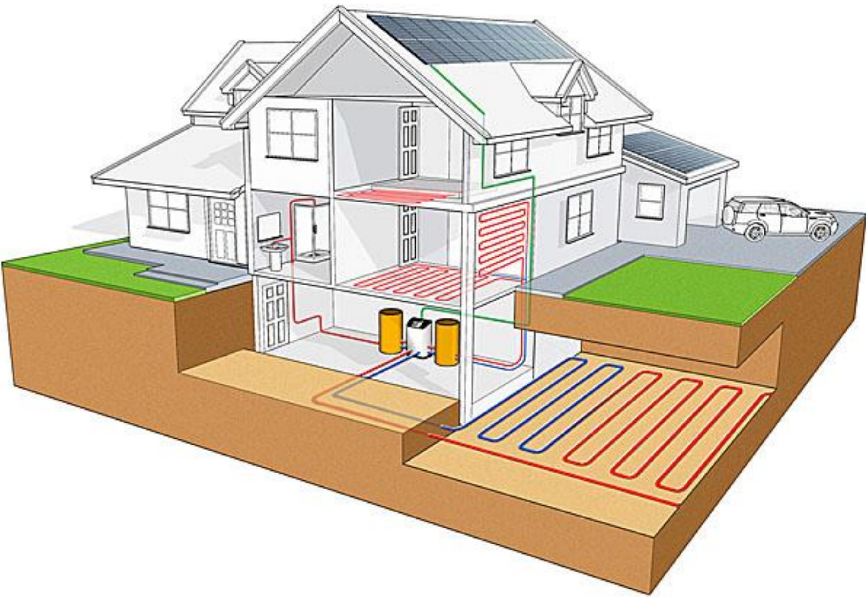
IMPIANTO A SONDE ORIZZONTALI
