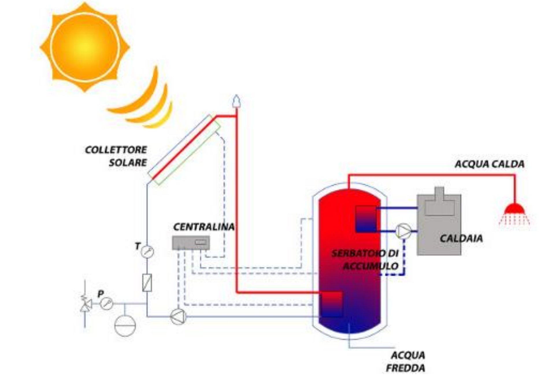
SCHEMA DI FUNZIONAMENTO
