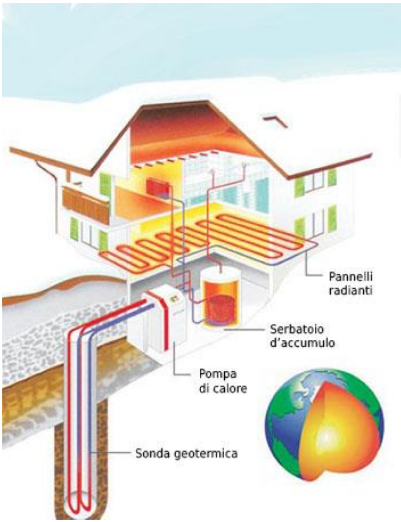
IMPIANTO A SONDE VERTICALI
